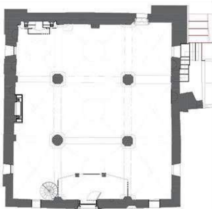
Pianta e prospetto stralciate dagli elaborati grafici del progetto
