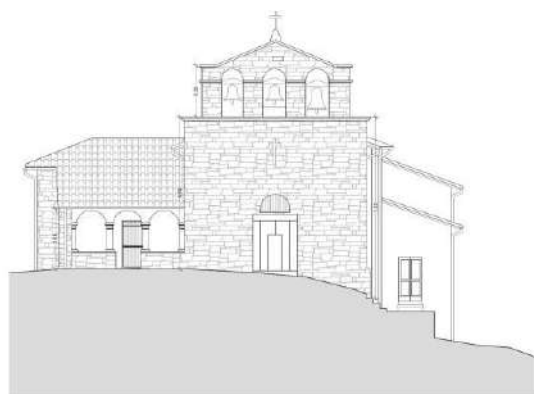
Prospetto EST
