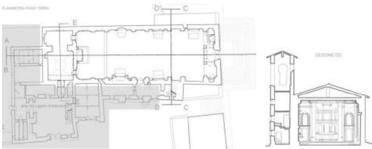
PIANTA PIANO TERRA E SEZIONE TRASVERSALE
