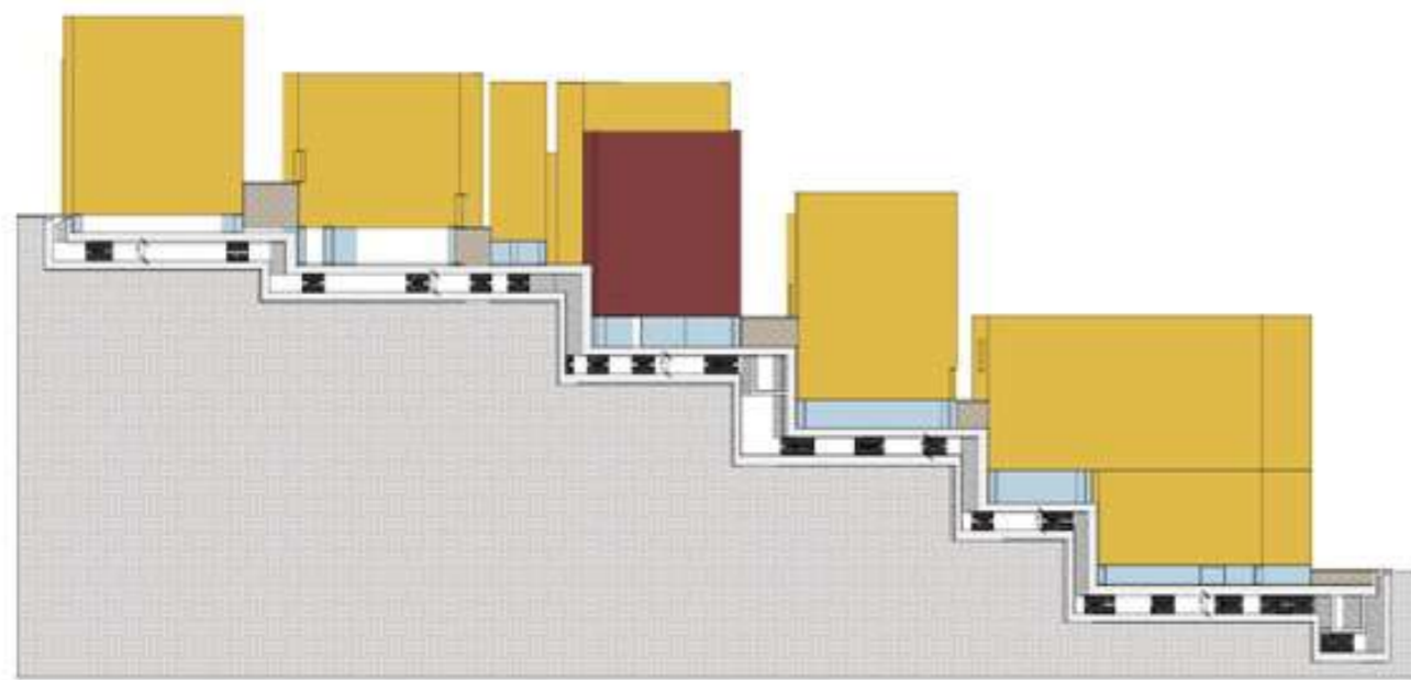
Figura 65. – Interventi di terrazzamento dei terreni e realizzazione dei sottoservizi: 1° contratto applicativo
