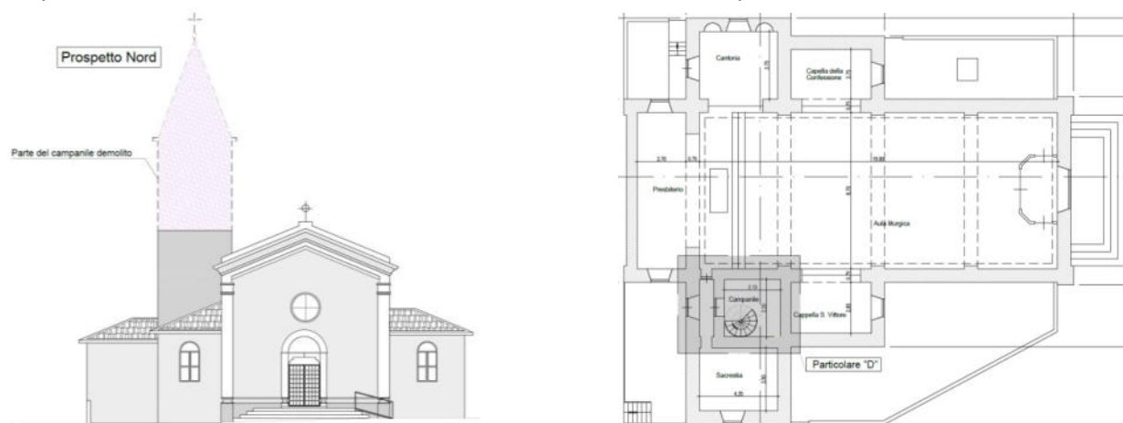
Pianta piano terra e prospetto principale
