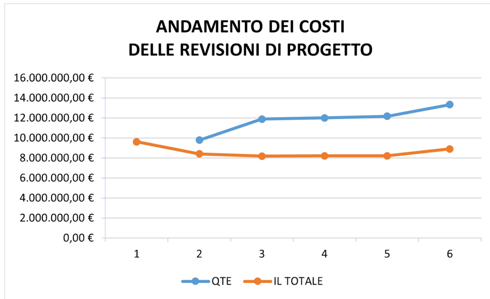
Fig. 4 - Andamento dei costi di intervento in relazione alle revisioni di progetto (in ascissa le revisioni di progetto ed in ordinata i relativi QTE e Importo Lavori) [QTE = Quadro tecnico economico; IL = Importo lavori].
