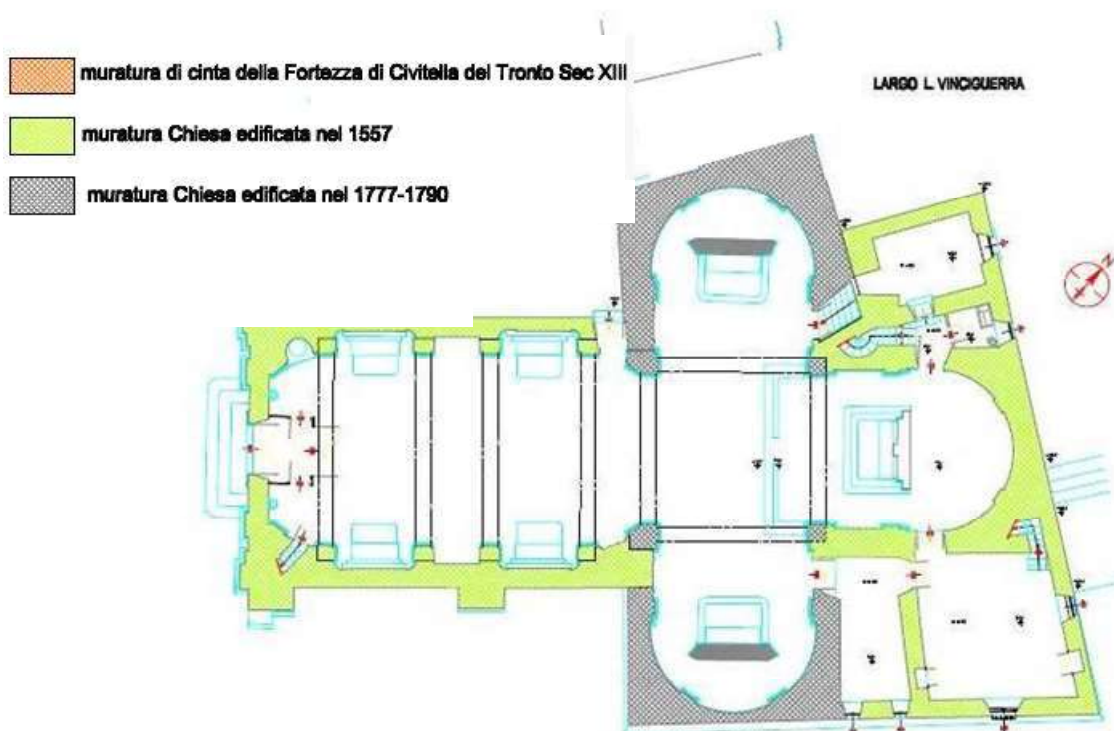
PIANTA PIANO TERRA - QUOTA +0.00m (vista dal basso verso l'alto)
