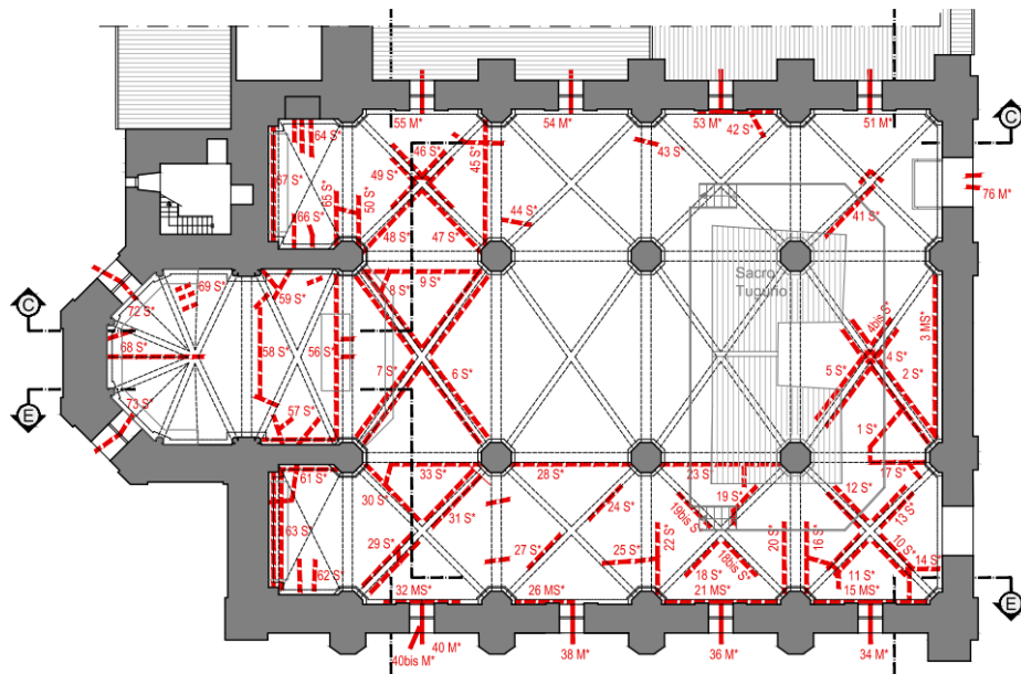
Quadro Fessurativo - Pianta delle murature e proiezione delle volte.
