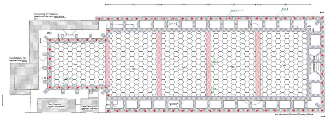
Chiesa di S. Lorenzo progetto della messa in opera delle nuove fondazioni.
